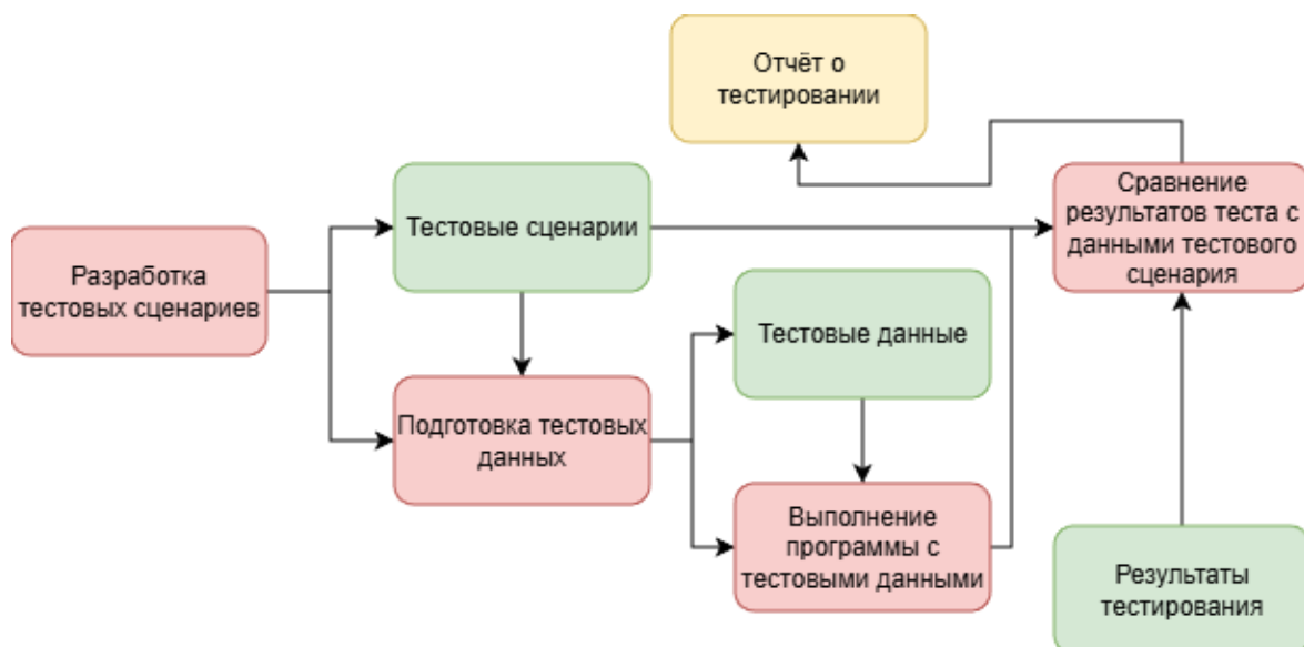
Рисунок 7 – Схема процесса тестирования
