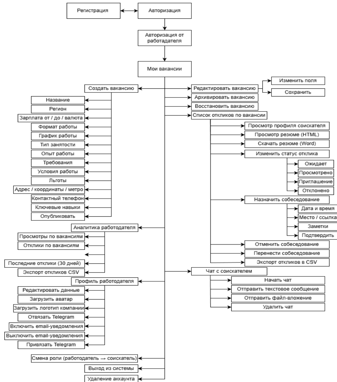
Рисунок 2 – Схема функционального тестирования работодателя в web-приложении JobFlex
