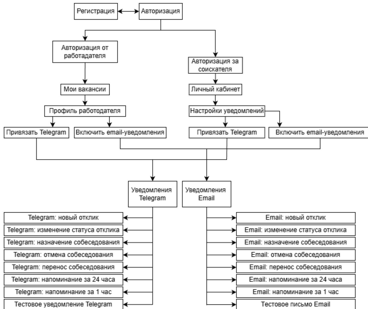
Рисунок 4 – Схема функционального тестирования уведомлений в web-приложении JobFlex
