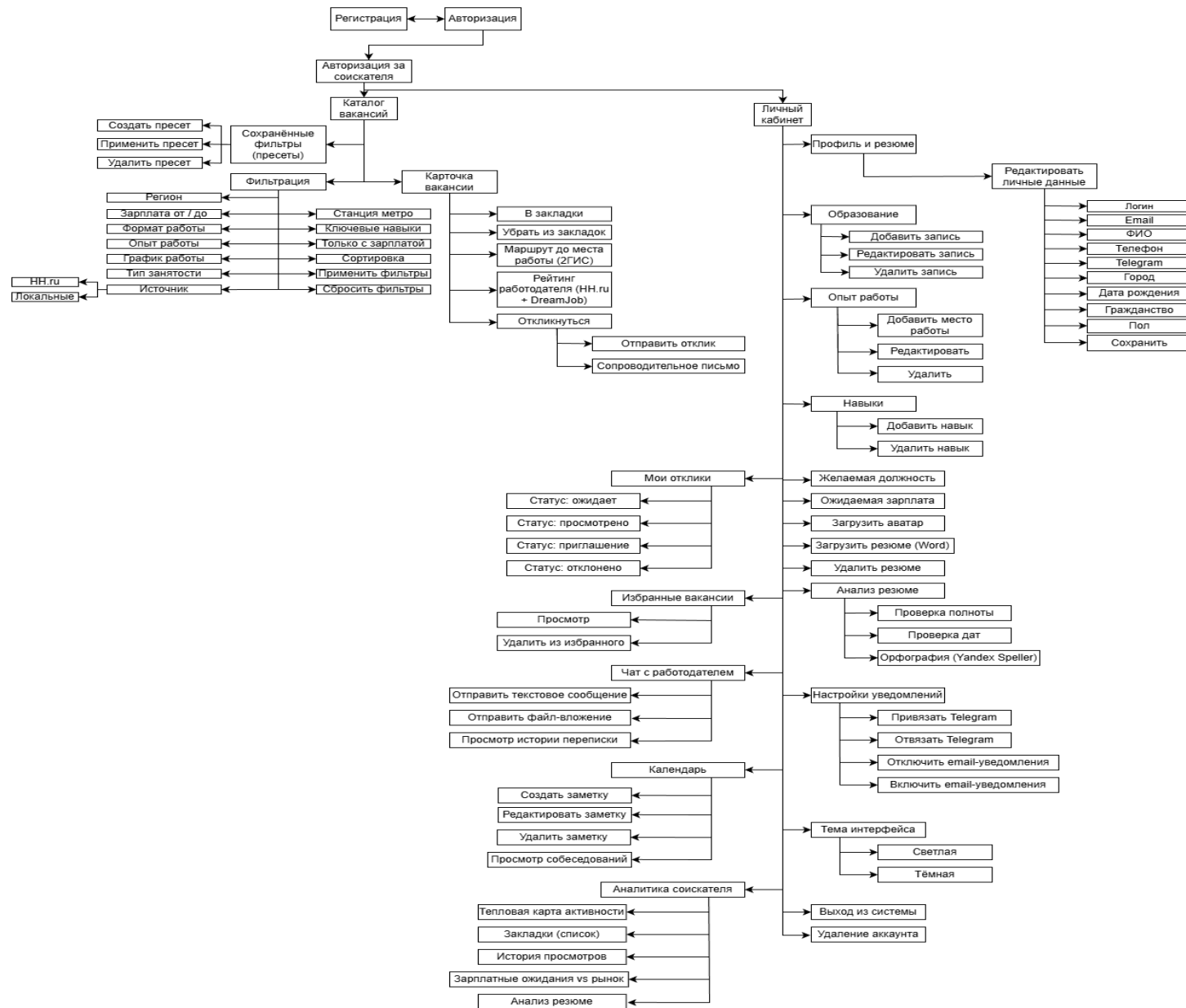
Рисунок 1 – Схема функционального тестирования соискателя в web-приложении JobFlex
