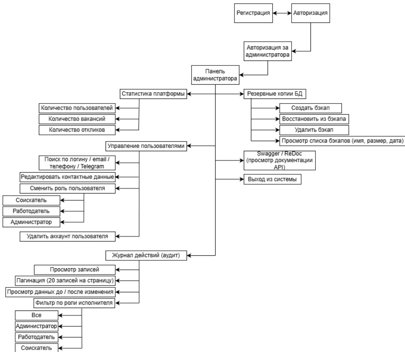
Рисунок 3 – Схема функционального тестирования администратора в web-приложении JobFlex
